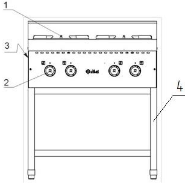
Рис. 1. Плита ПГК-49П-П-А
