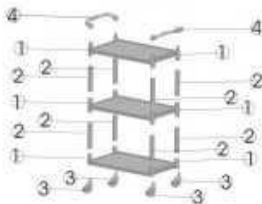
Чертеж сборки
