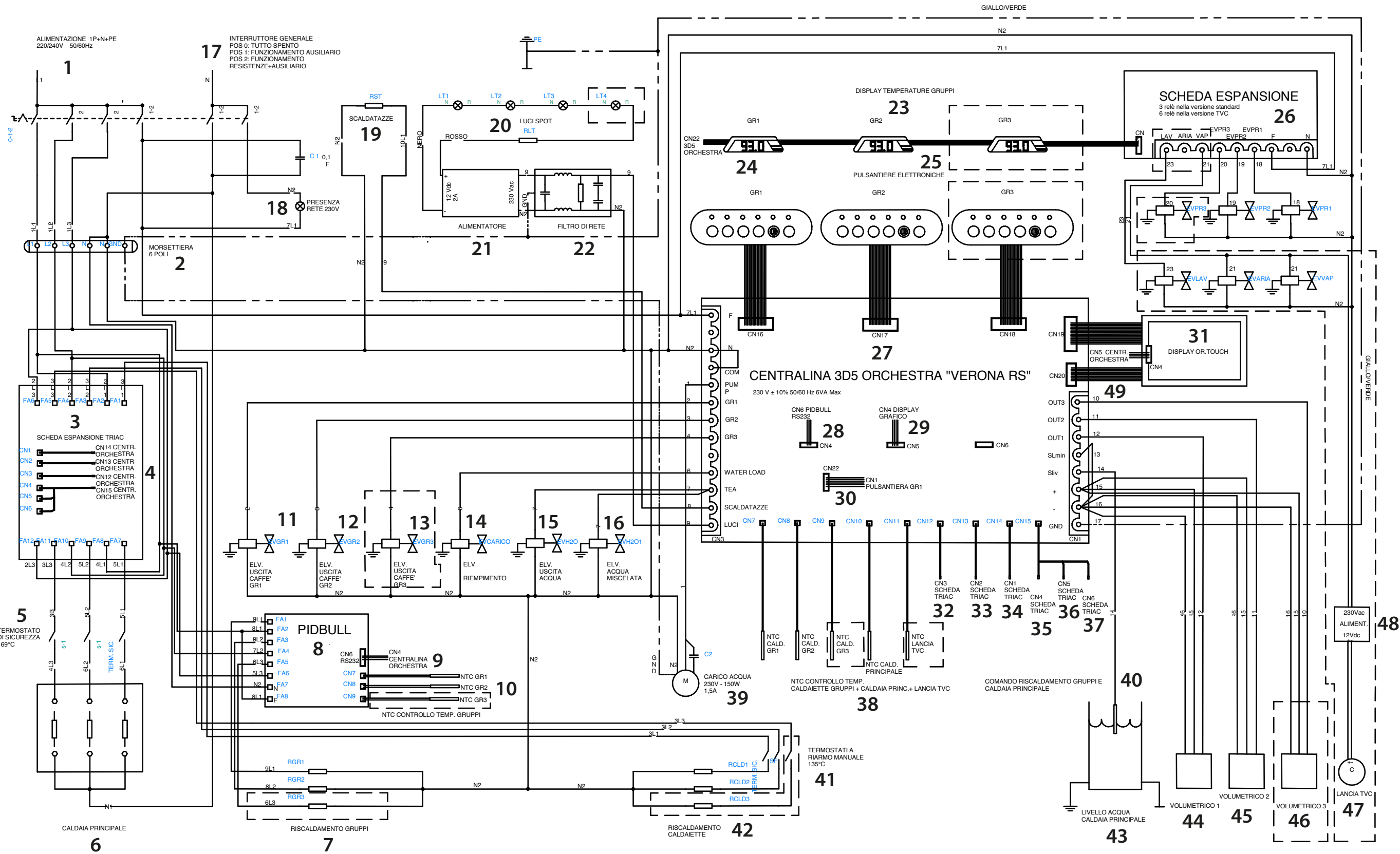
SCHEMA ELETTRICO VERONA RS 2-3GR SED TCS ACQ.MISC. TVC LUCI
